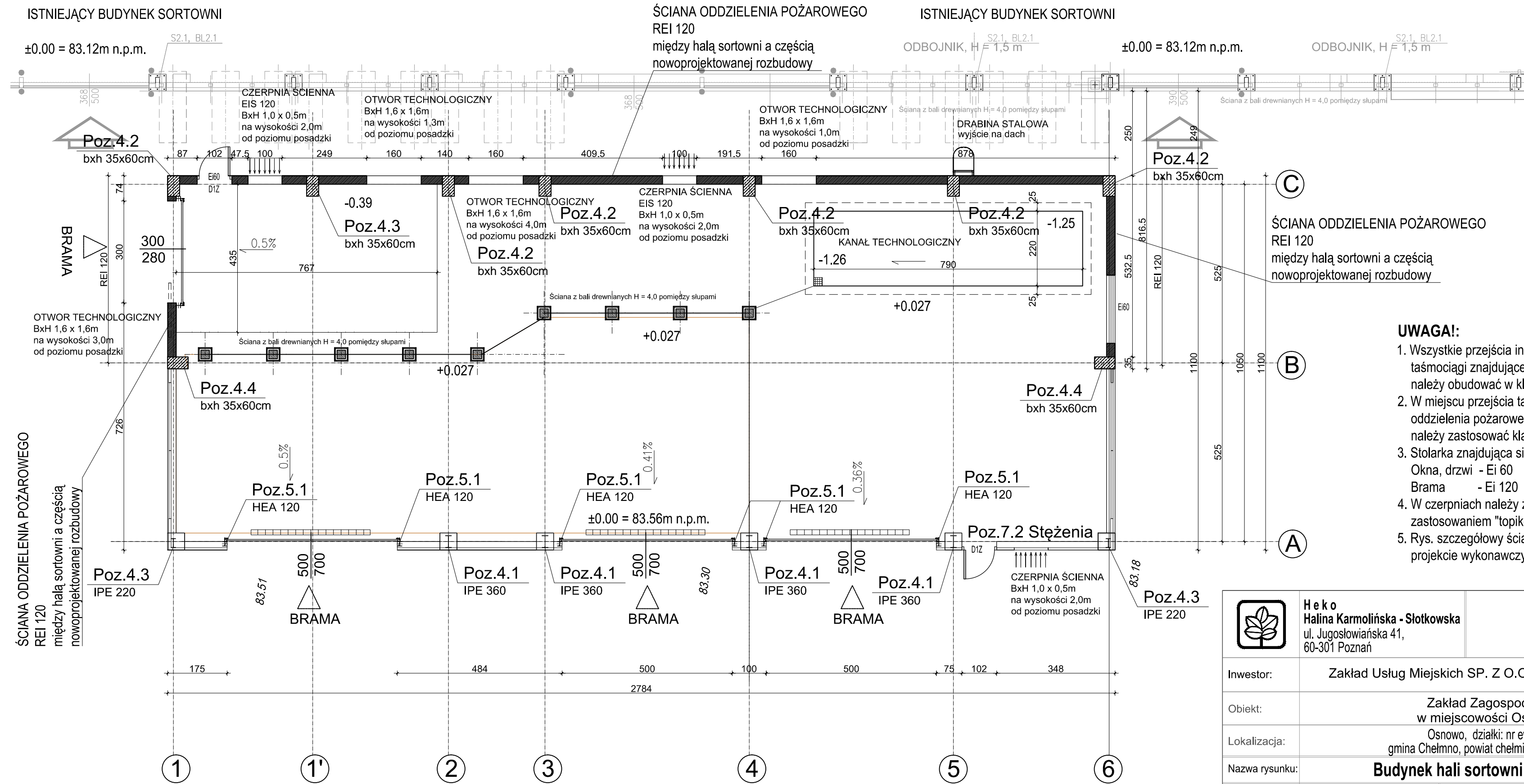
RZUT KONSTRUKCJI HALI SORTOWNI NA POZ.±0,00 1:100
